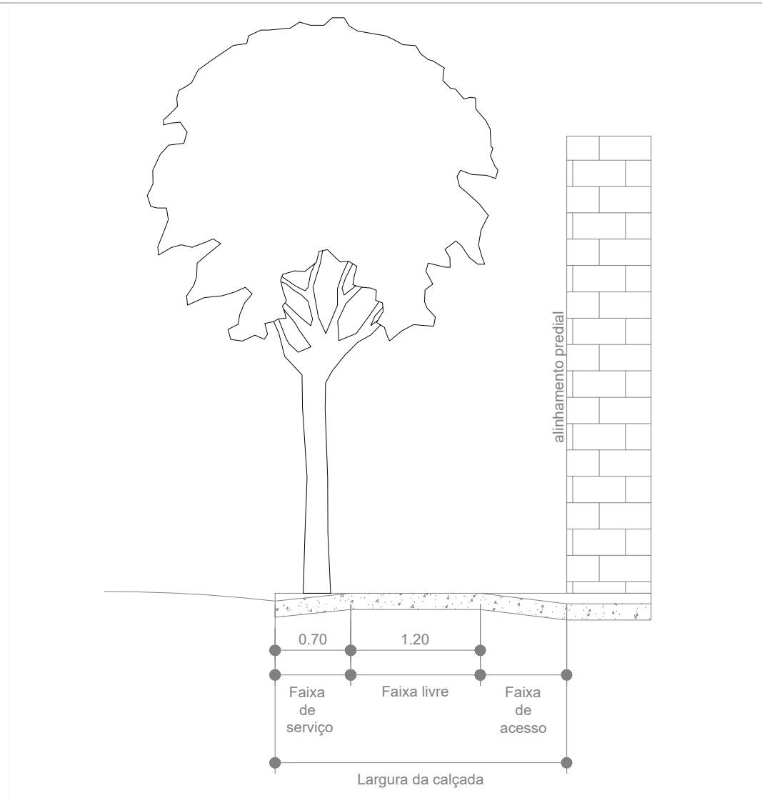
DETALHE ACESSO VEÍCULOS - CORTE SEM ESCALA
