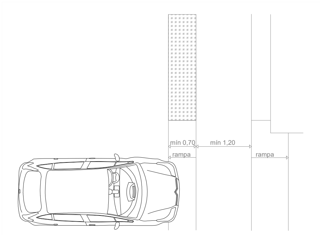
DETALHE ACESSO VEÍCULOS - PLANTA SEM ESCALA
