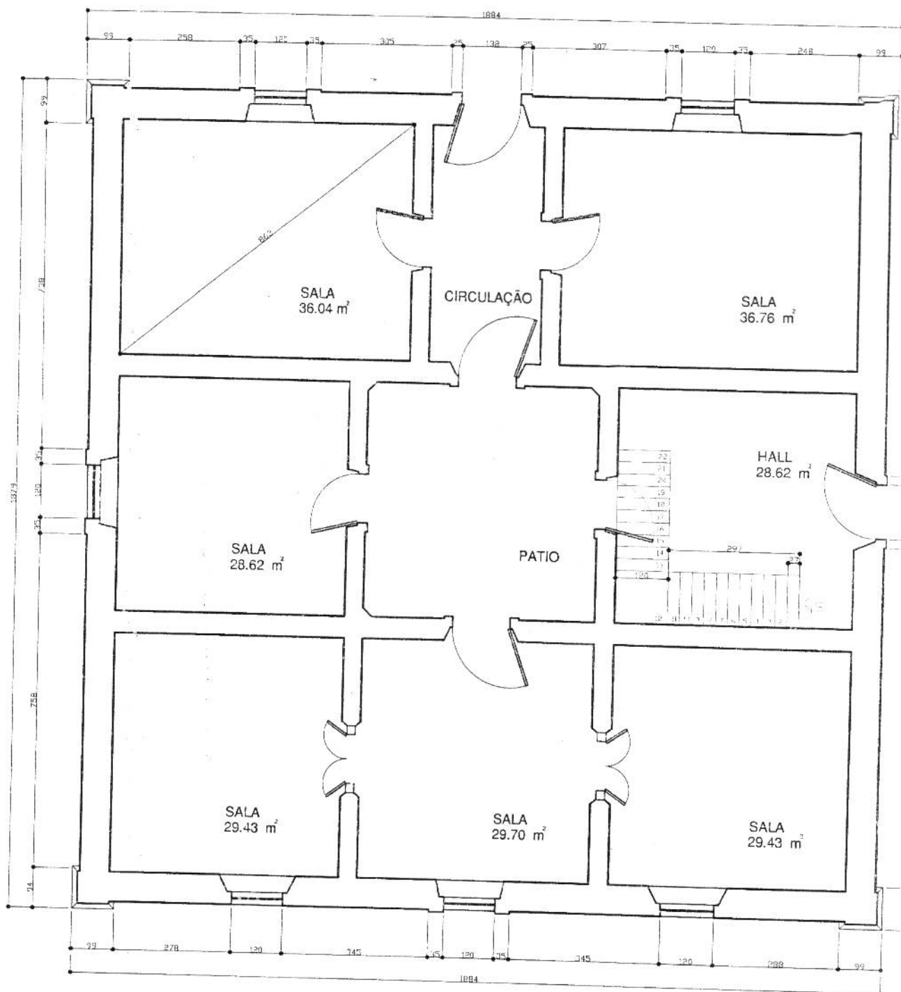
PLANTA PRIMEIRO PAVIMENTO ho ESC.: 1/100
